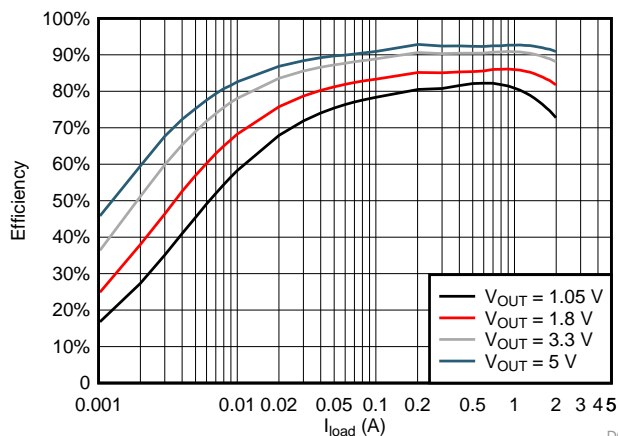
TPS563201 效率
