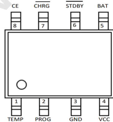
ESOP-8封装 (底部带有散热片需接地)
